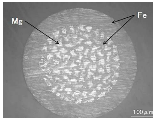
Mg/Feクラッド細線 φ0.5mm
