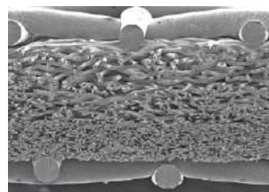
ろ材断面
