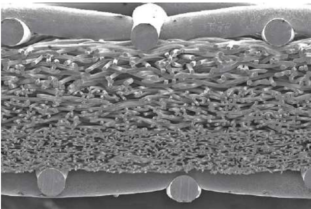
ろ材断面
