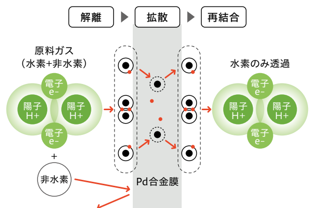
水素透過のメカニズム
