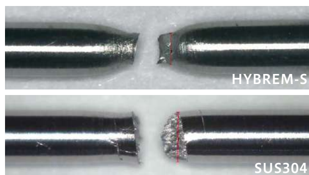
低温SSRT試験後の破断部の比較 (破断部が大きい=脆化によって延性が低下していることを示す)
